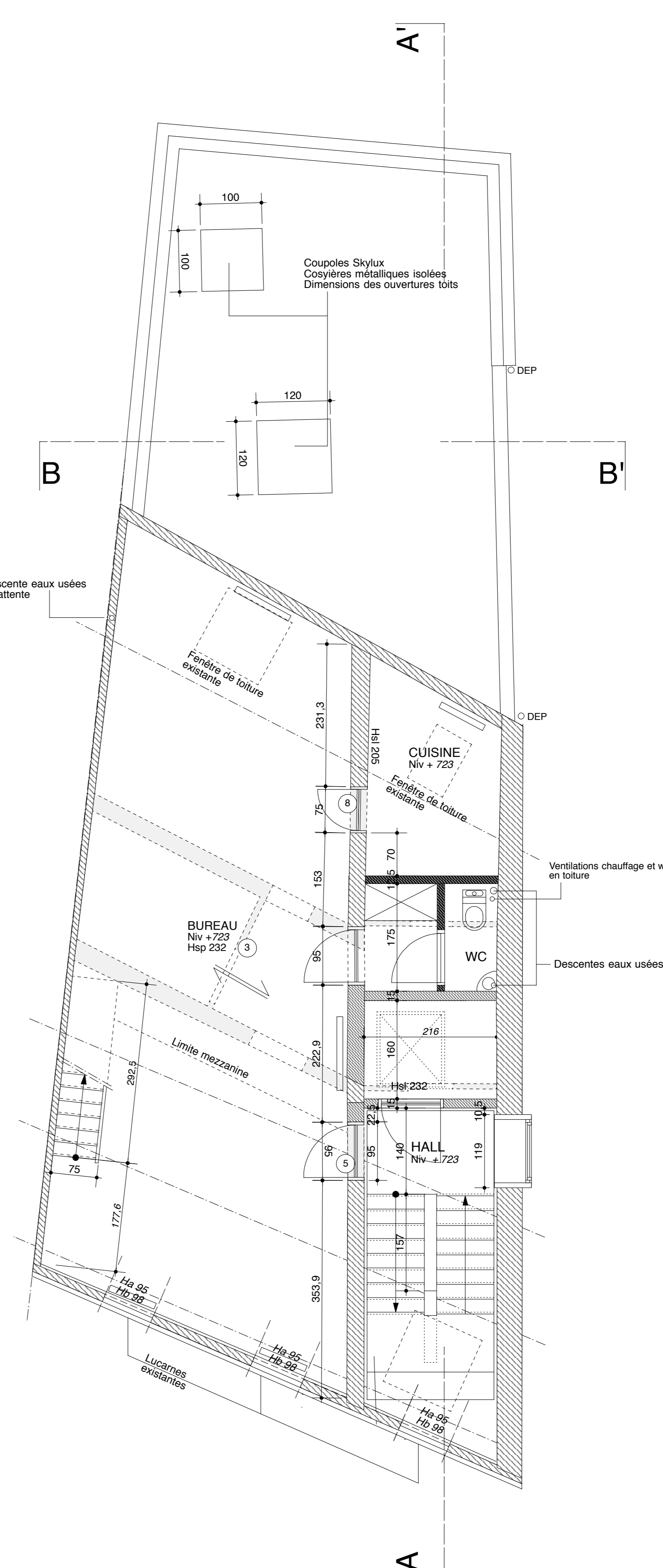
PLAN DU 2ème ETAGE
