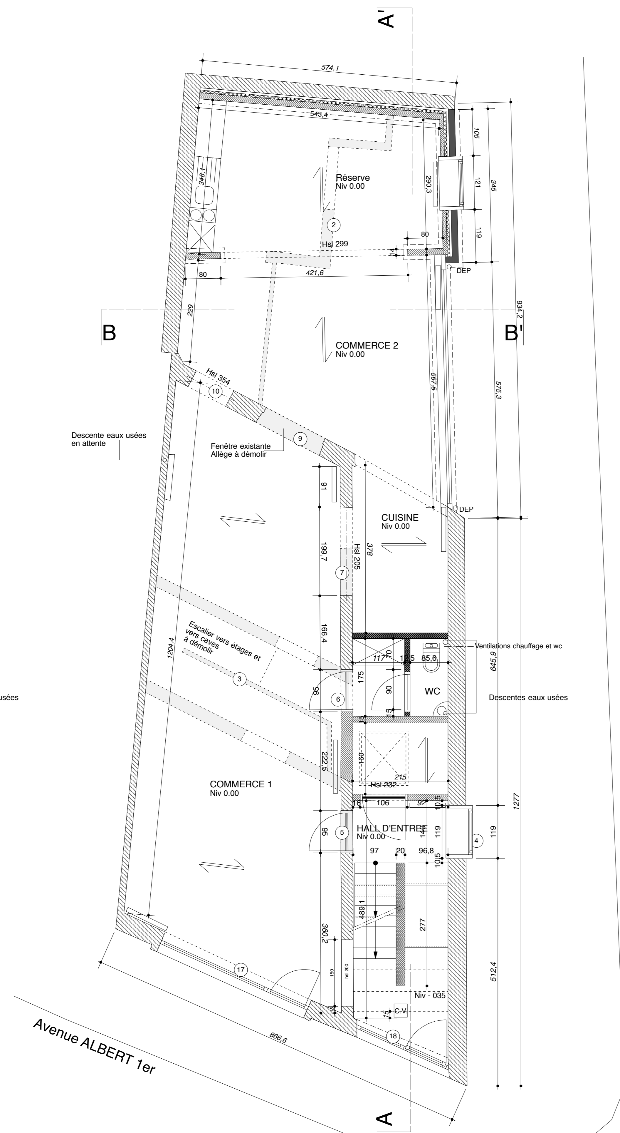
PLAN DU REZ-DE-CHAUSSEE
