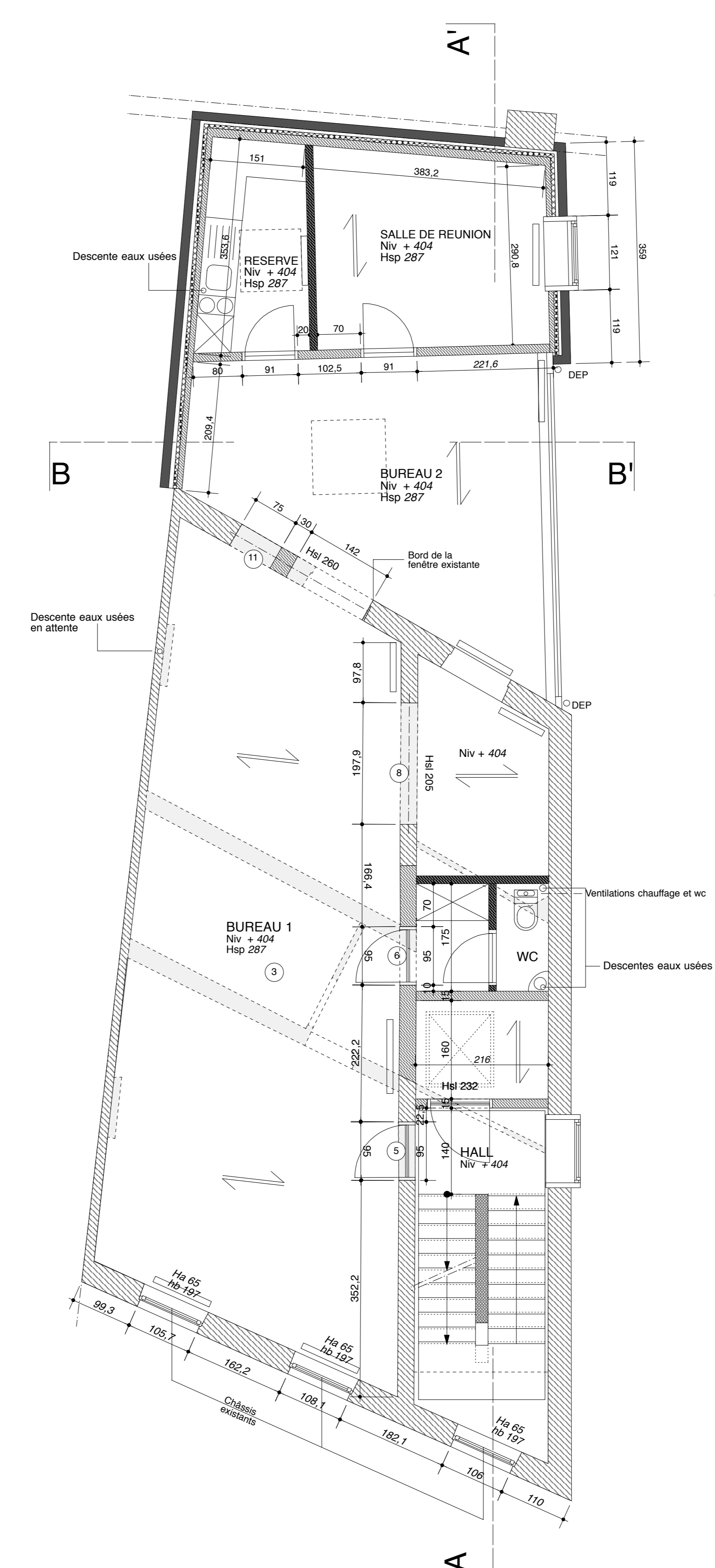
PLAN DU 1er ETAGE
