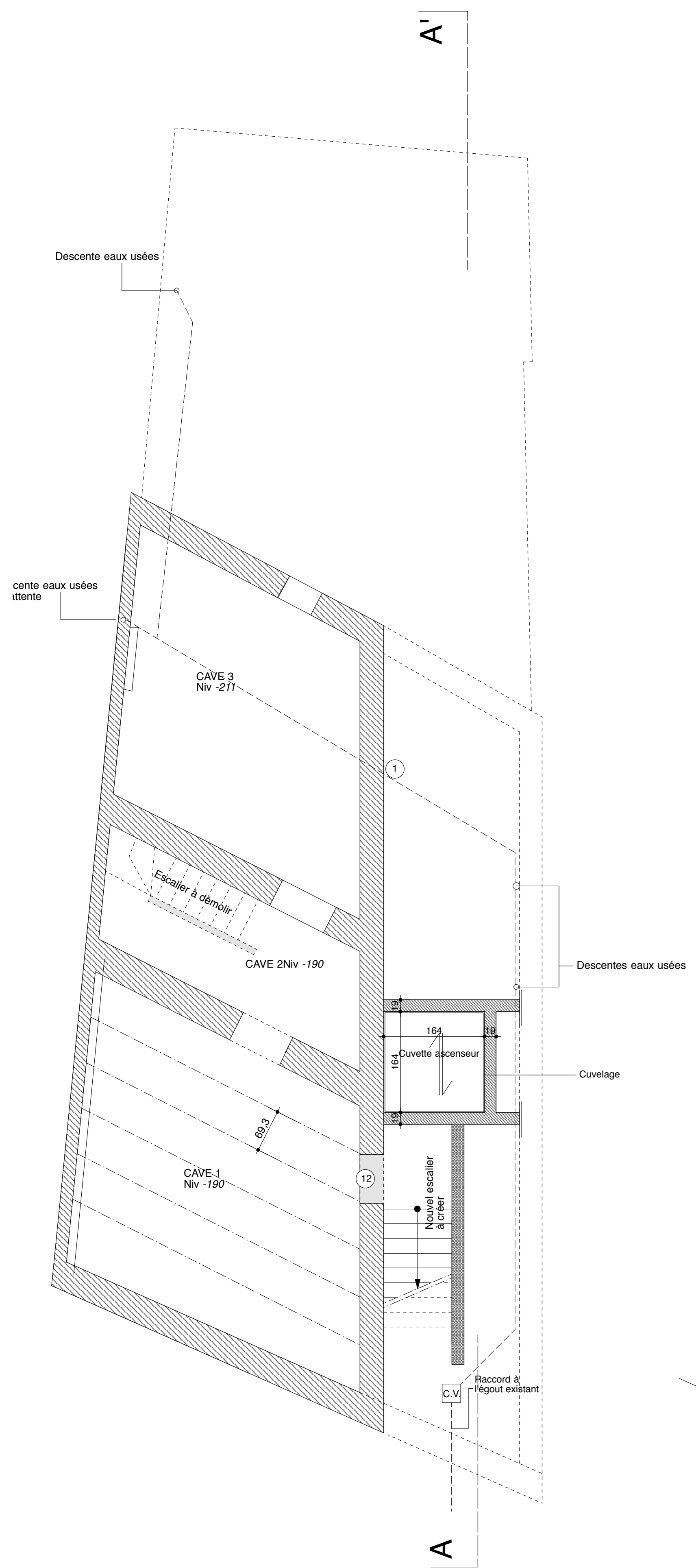
PLAN DU SOUS-SOL
