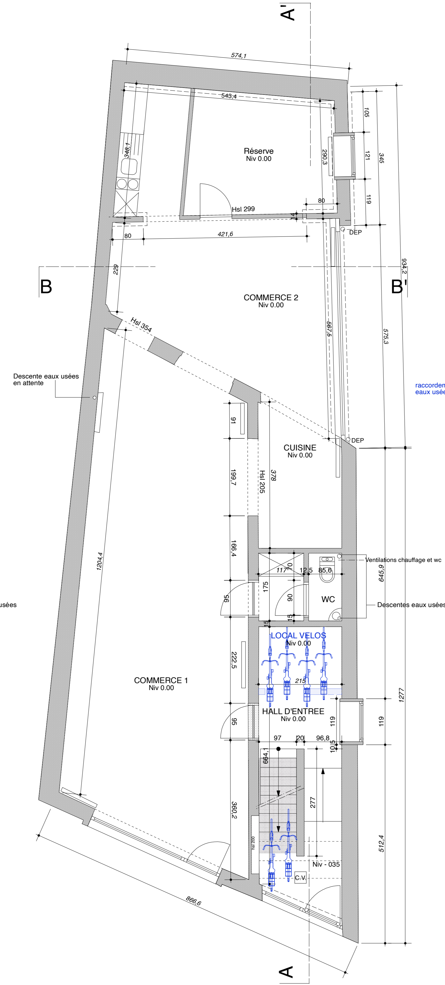
PLAN DU REZ-DE-CHAUSSEE
