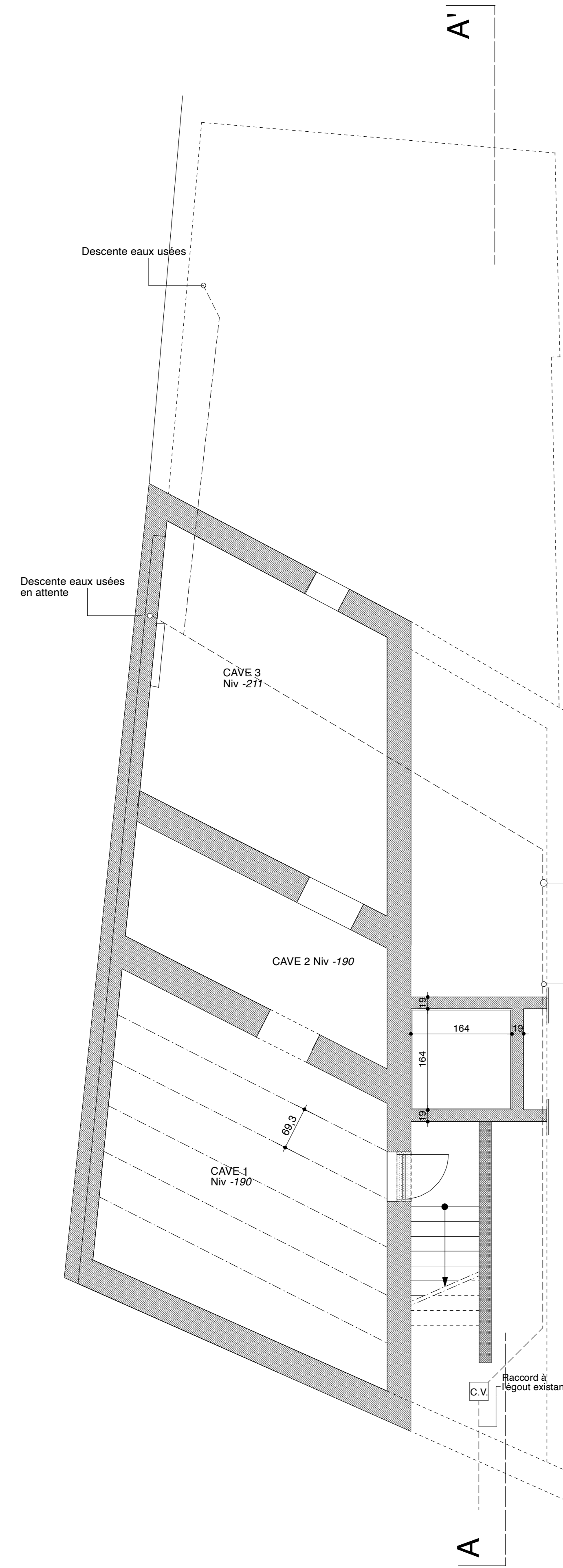
PLAN DU SOUS-SOL
