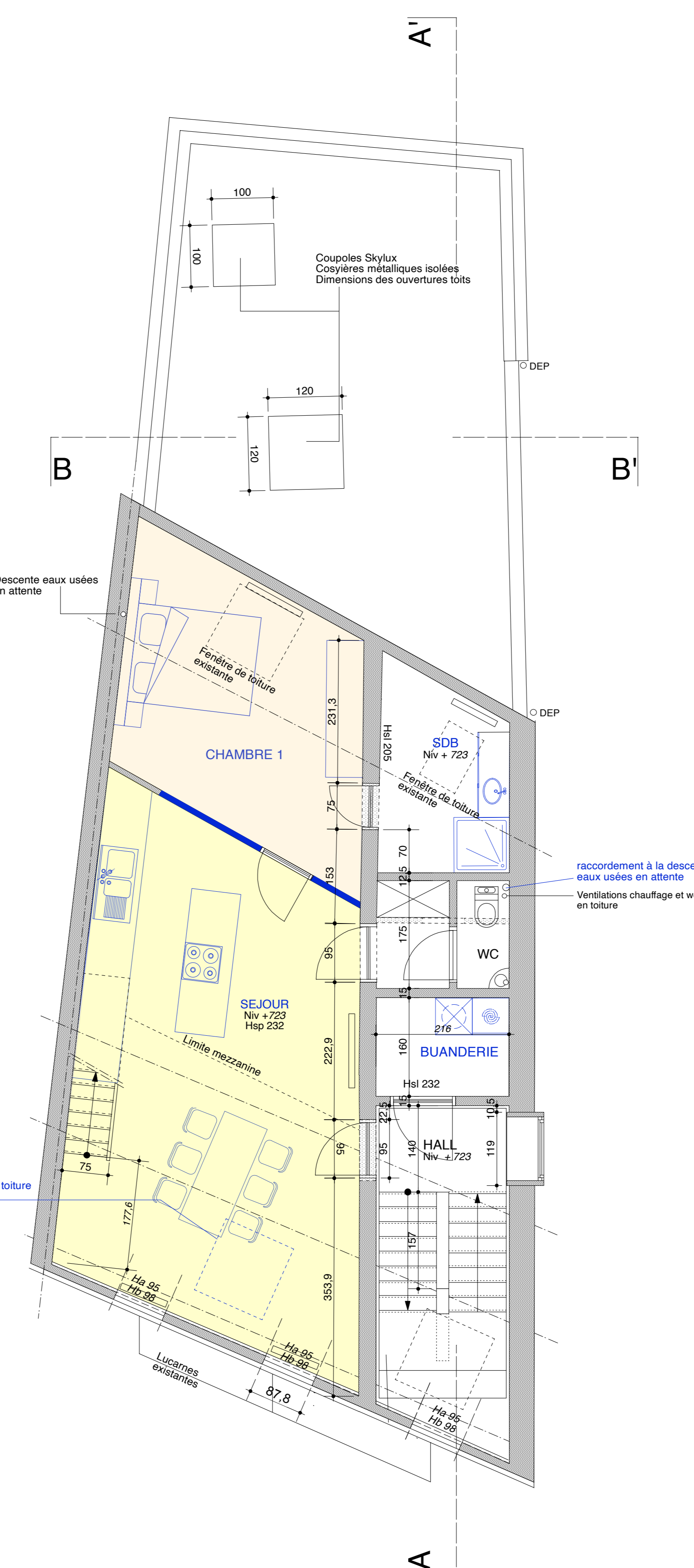
PLAN DU 2ème ETAGE
